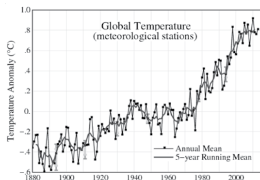
Figur 1. Den årlige globale middeltemperaturen i den lavere atmosfæren 1880-2014. Den svarte kurva viser hvor mye den faktiske temperaturen i gjennomsnitt over året avviker fra middeltemperaturen for perioden 1951-1980. Den røde kurva viser for hvert år gjennomsnittet for det året og de to foregående og de to etterfølgende åra. Den jevner ut variasjonene i været fra det ene året til det neste og framhever den langsiktige tendensen.
