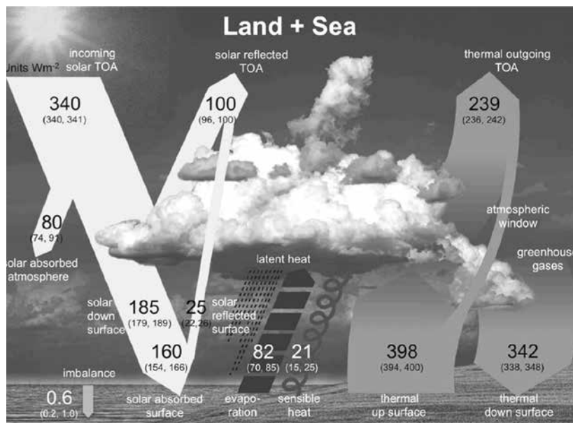
Figur 4. Jordas energiregnskap [11]. Pilene viser energistrømmene inn og ut av Jorda og hvordan den innkommende energien fordeles seg. Alle energistrømmene er uttrykt i watt pr kvadratmeter (energimengde pr sekund pr kvm).
