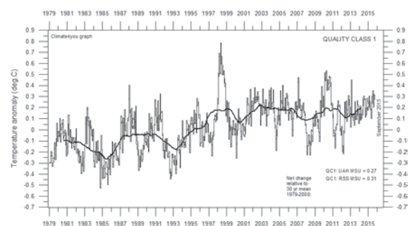
Figur 2. Den månedlige globale middeltemperaturen i den lavere atmosfæren 1979-2015. Den blå kurva viser avviket fra middeltemperaturen for perioden 1979-2008. Den svarte kurva representerer gjennomsnittet over 37 måneder (fra og med 18 måneder før til og med 18 måneder etter).
