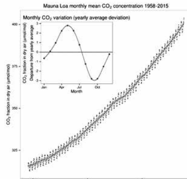
Figur 3. Til venstre: årlige globale utslipp av CO 2 til atmosfæren 1965-2011 [6]. Til høyre: midlere konsentrasjon av CO 2 i atmosfæren 1958-2015 [7].
