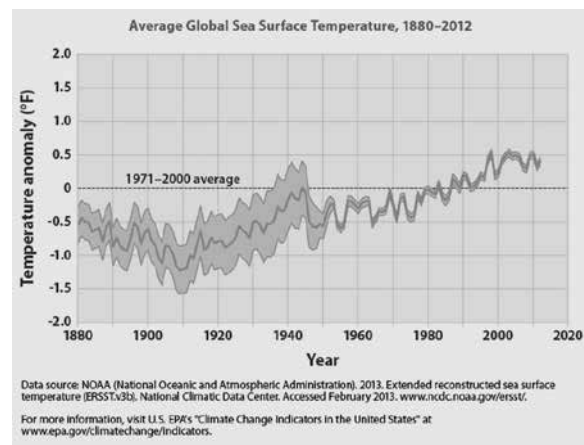
Figur 5. Slik har gjennomsnittstemperaturen i overflatevannet i verdenshavene utvikla seg siden 1880 [12].
