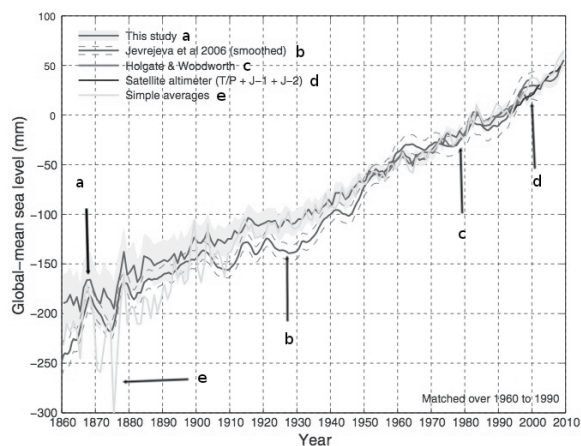
Figur 6. Økinga av havnivået 1860-2010 [13]. De tre kulørte kurvene stammer fra tre ulike artikler og metoder.
