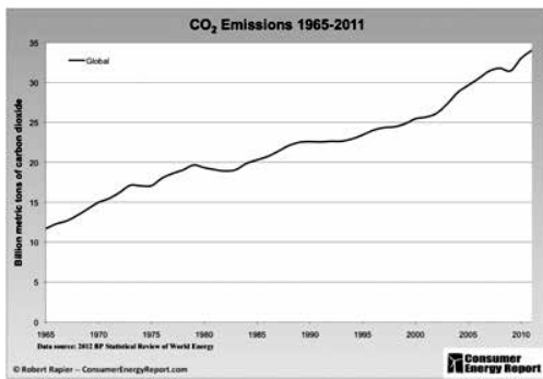
Figur 3. Til venstre: årlige globale utslipp av CO 2 til atmosfæren 1965-2011 [6]. Til høyre: midlere konsentrasjon av CO 2 i atmosfæren 1958-2015 [7].
